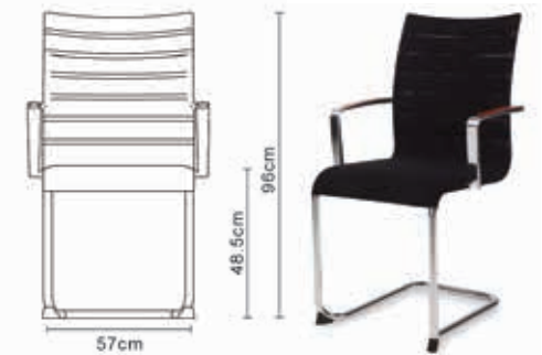
05/1A Depth 60cm Weight 9.3kg
